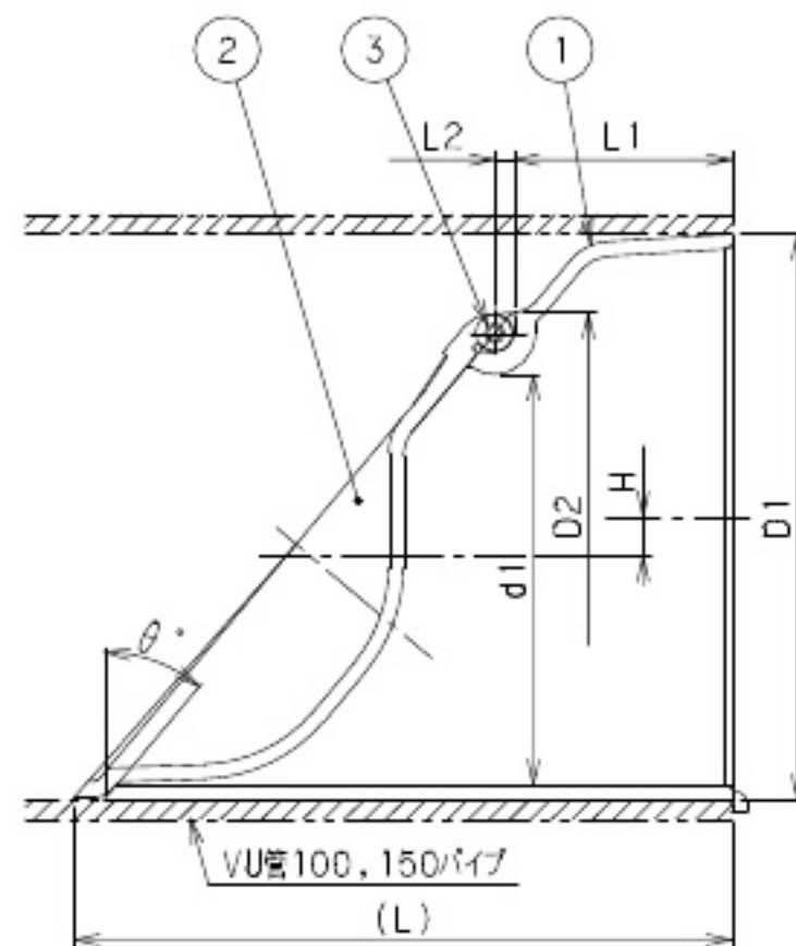
VU管：呼び径100, 150
