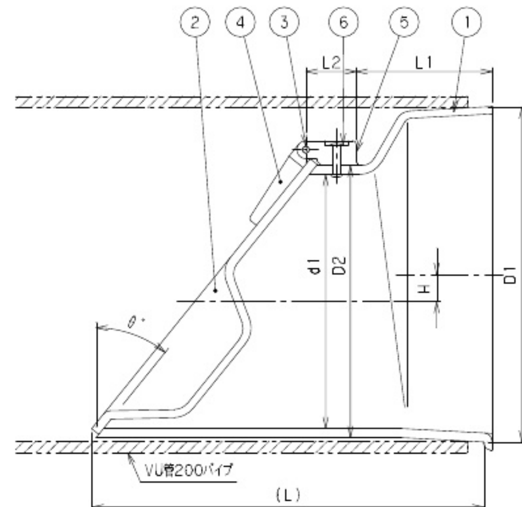
VU管：呼び径200
