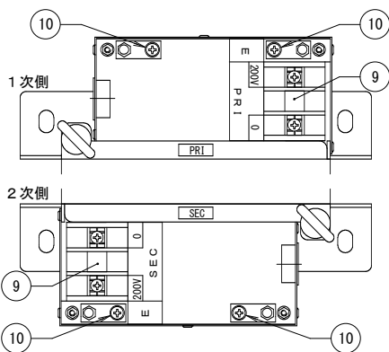
端子箱蓋 解放圖
