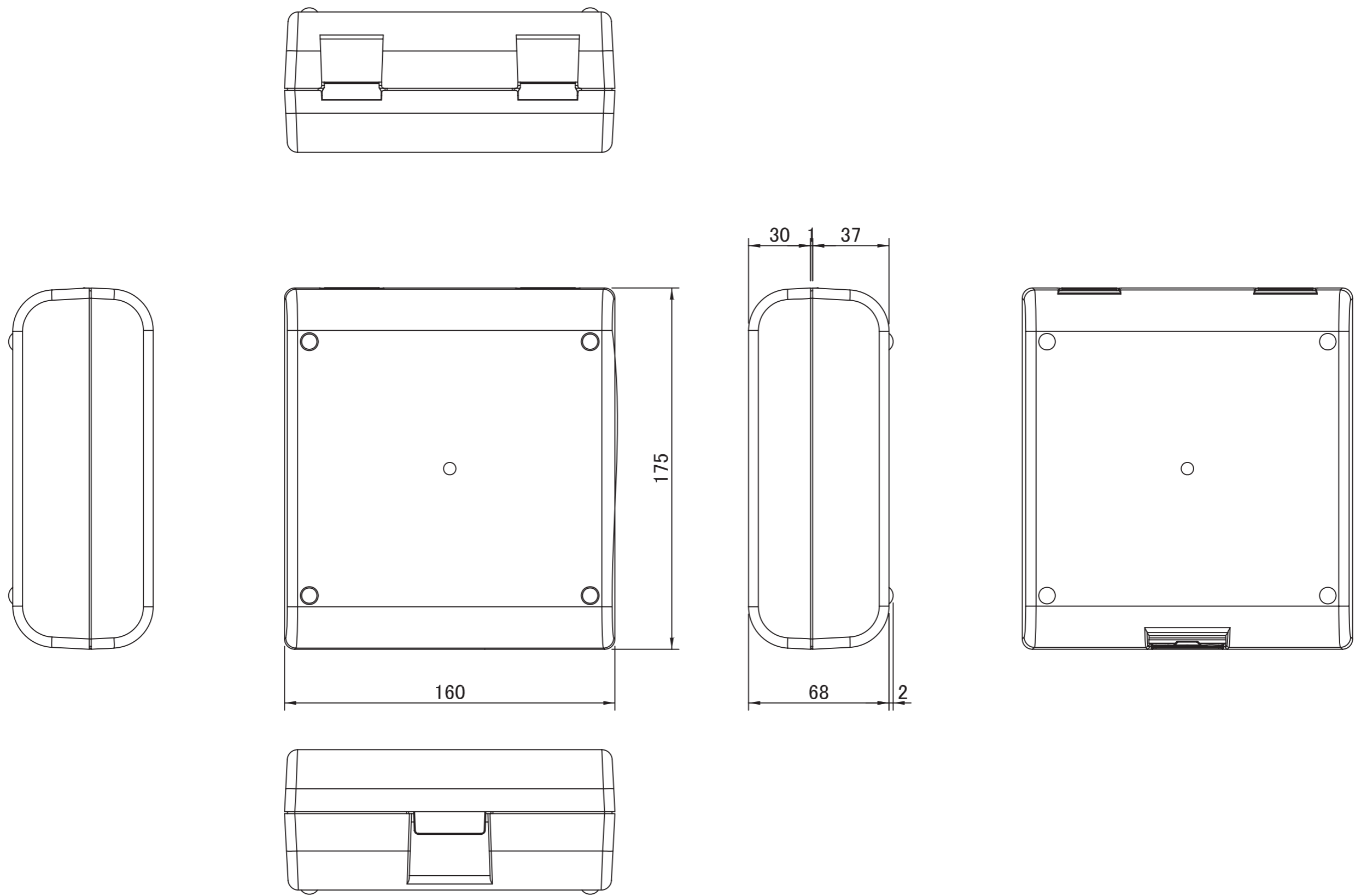
HT-120付属ケース 外形寸法図
