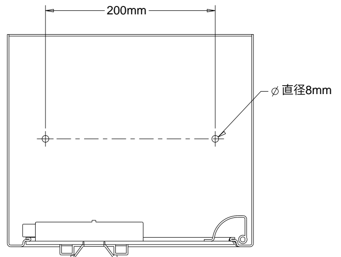
【底面図】
