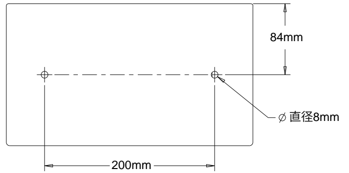
【背面図】
