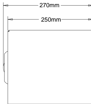
【側面図】
