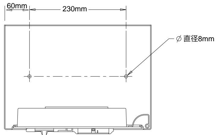
【底面図】
