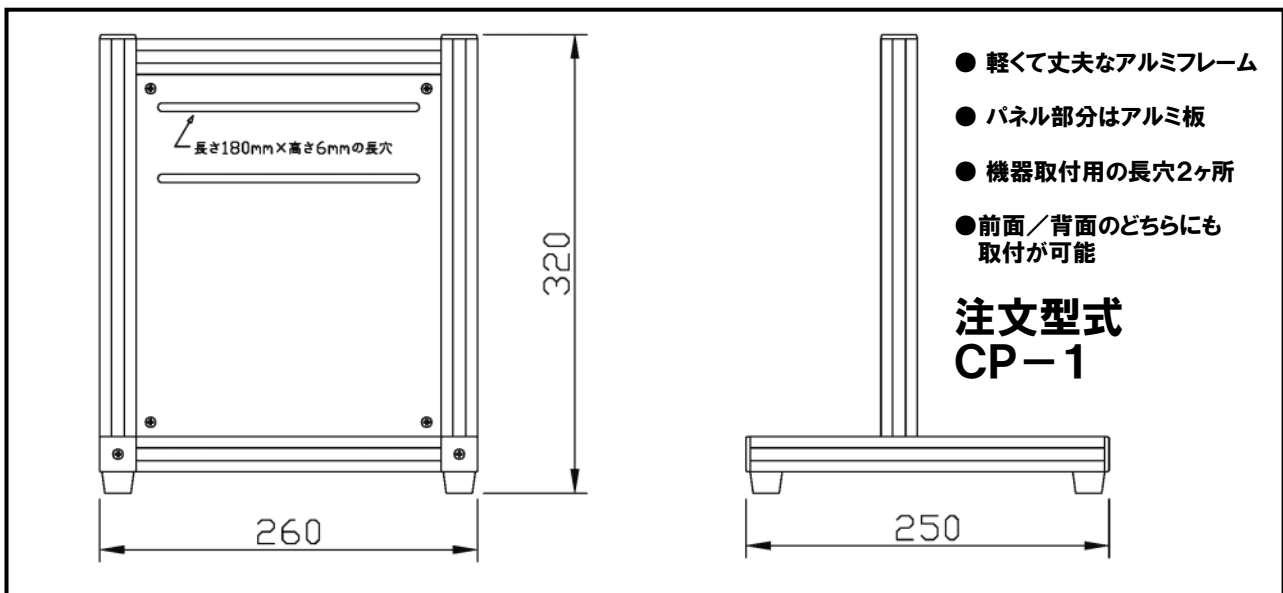
■CPクリーンパネルの外形図
