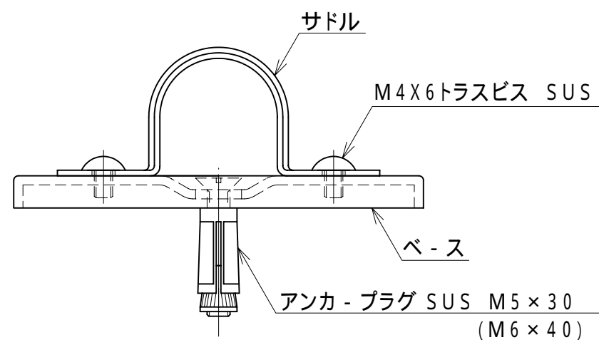
組立図
