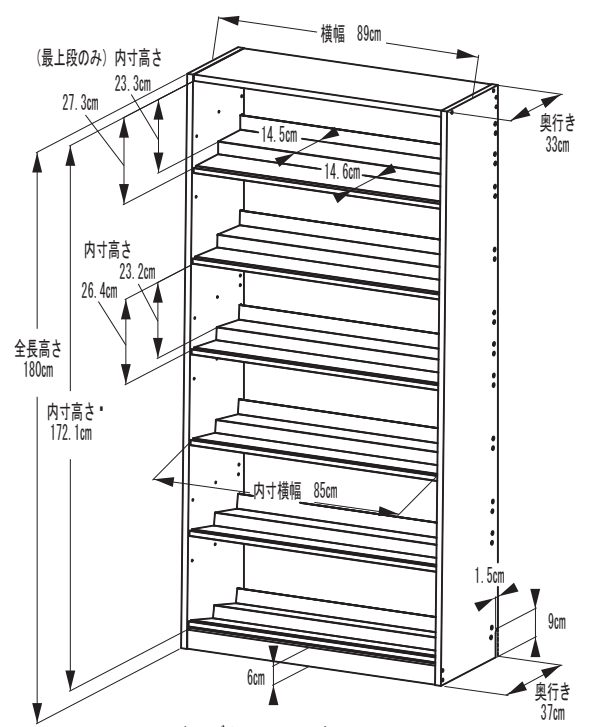
タンDEMCDストッカー TCS 890 棚6段段設定時
