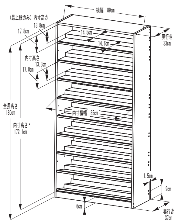
タンDEMCDストッカー TCS 890 棚9段段設定時
