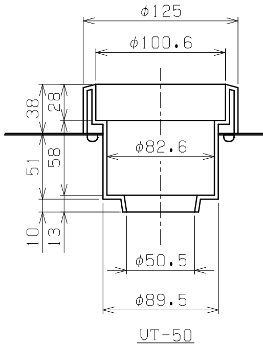
ツーリングホルダー取付 詳細
