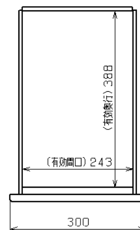
引出し詳細
