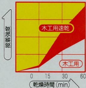
木工用接着剤スピード比較
