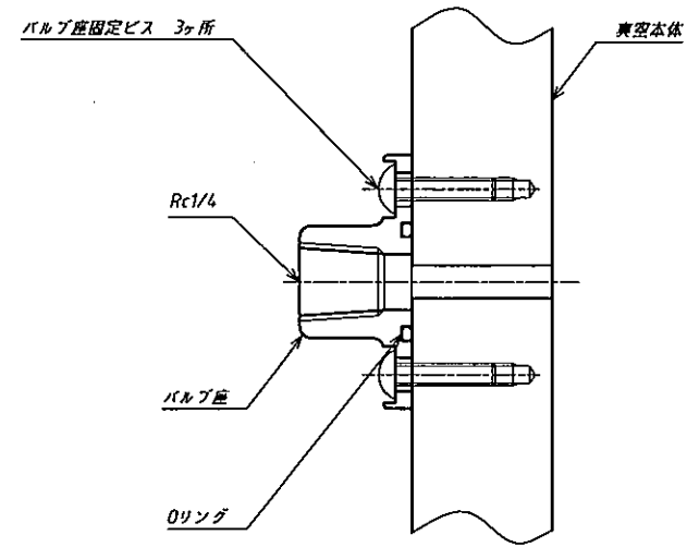
バルブ座取付参考図
