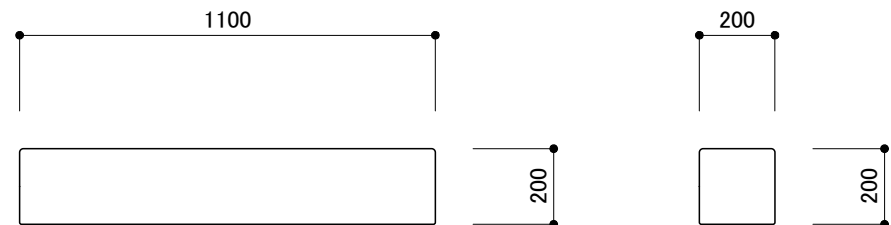
ベンチ KS-D200-BC1100
