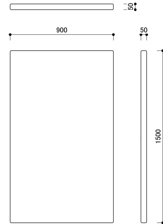
壁パネル900 KS-SQ-WP900
