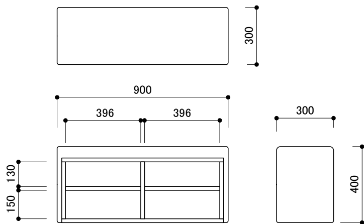
シューズベンチ KS-D300-SB
