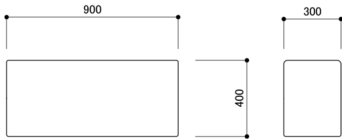
W900ベンチ KS-D300-BC900
