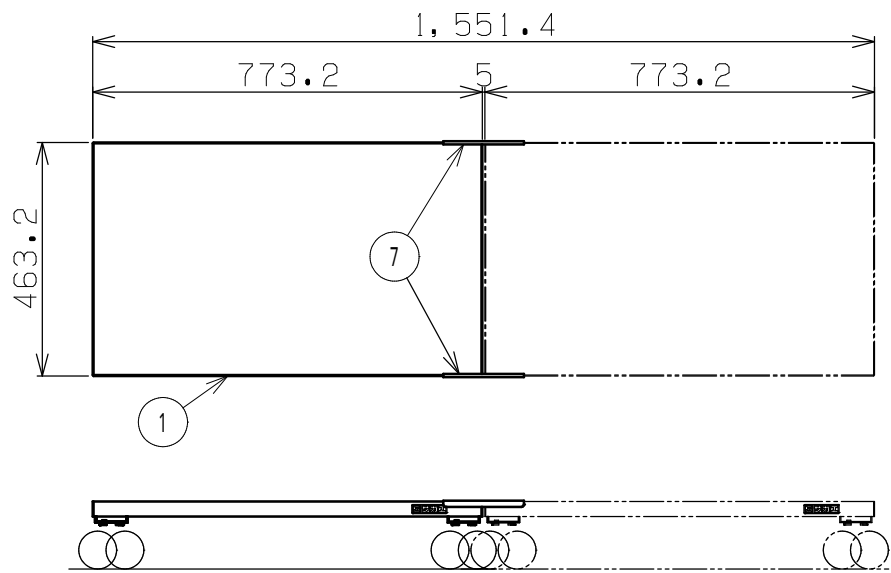
下部連結金具
