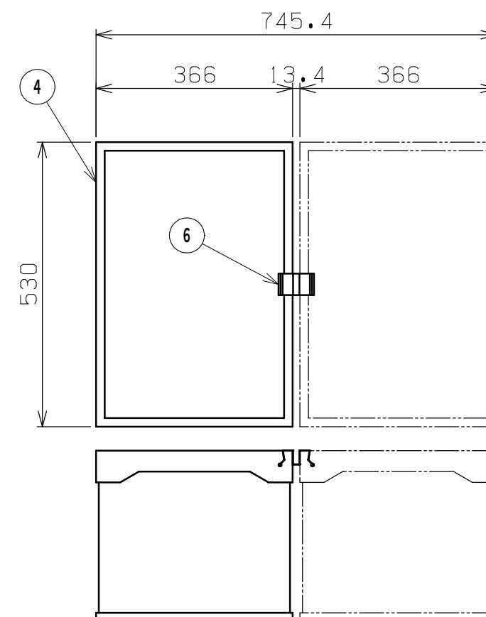
上部連結金具
