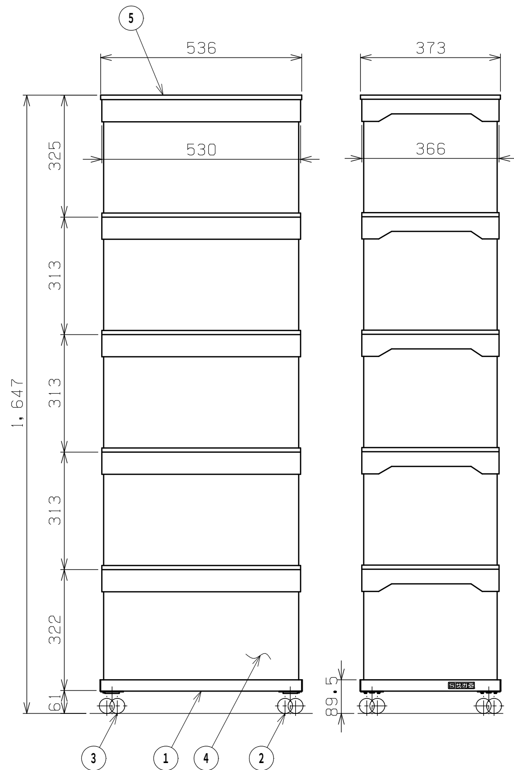
コンテナ、組立時
