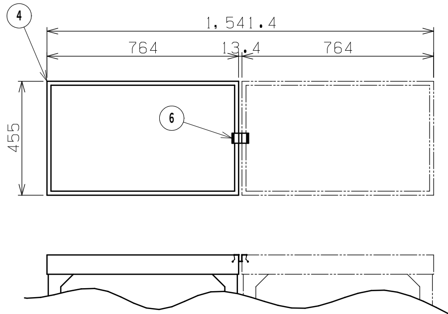
上部連結金具
