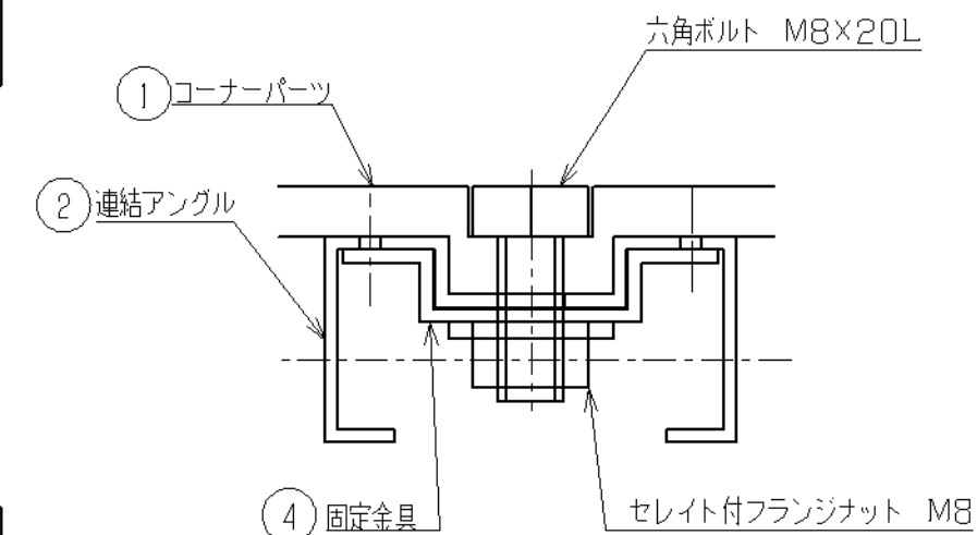
矢視 A-A
