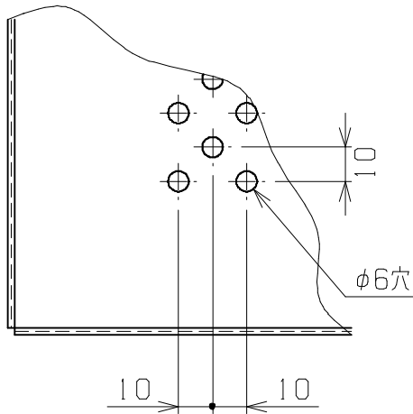
パンチングメタル詳細 (S=1:2)
