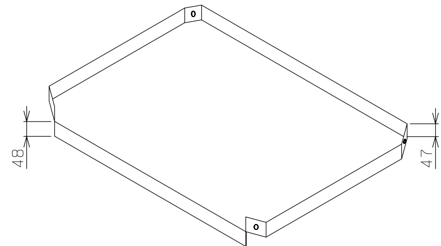
3方コボレ止め棚板 詳細図
