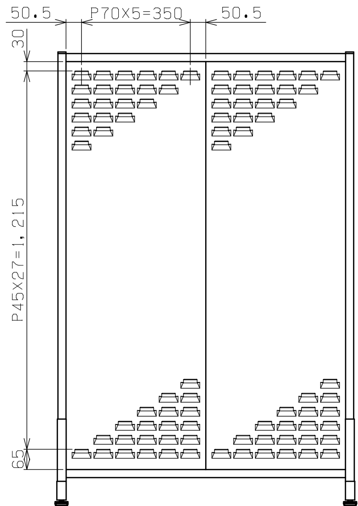
取付部詳細 S=1:12
