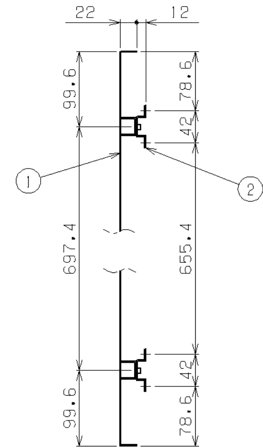
組付詳細 (S=1/5)
