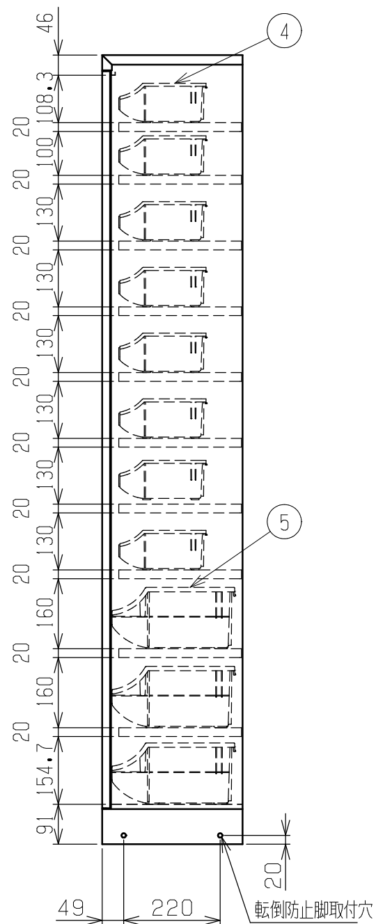
本体塗装色 パーツボックス 品 番 サカエホワイト アイボリー Z-1NR (レッド) ... 18個 SCR-18CDI Z-1NY (イエロー) ... 12個 Z-1NB (ブルー) ... 18個 Z-2NR (レッド) ... 4個 Z-2NY (イエロー) ... 4個 Z-2NB (ブルー) ... 4個
