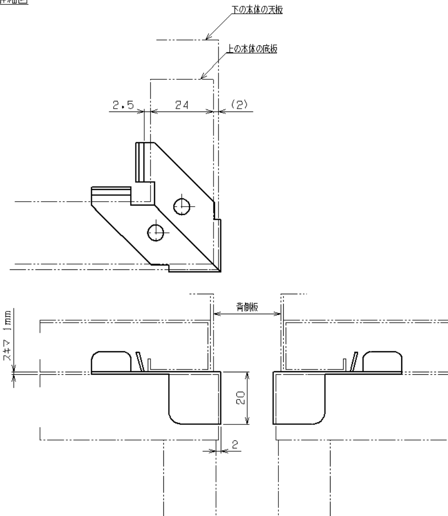
取付詳細図
