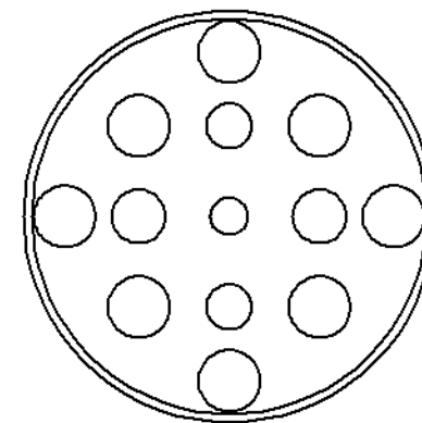
矢視A
