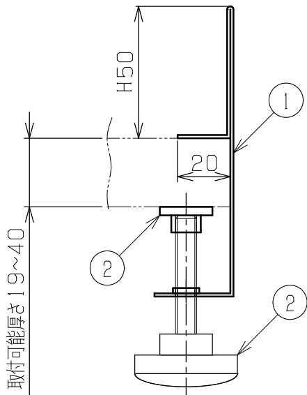
天板取付詳細 (S=1:2)
