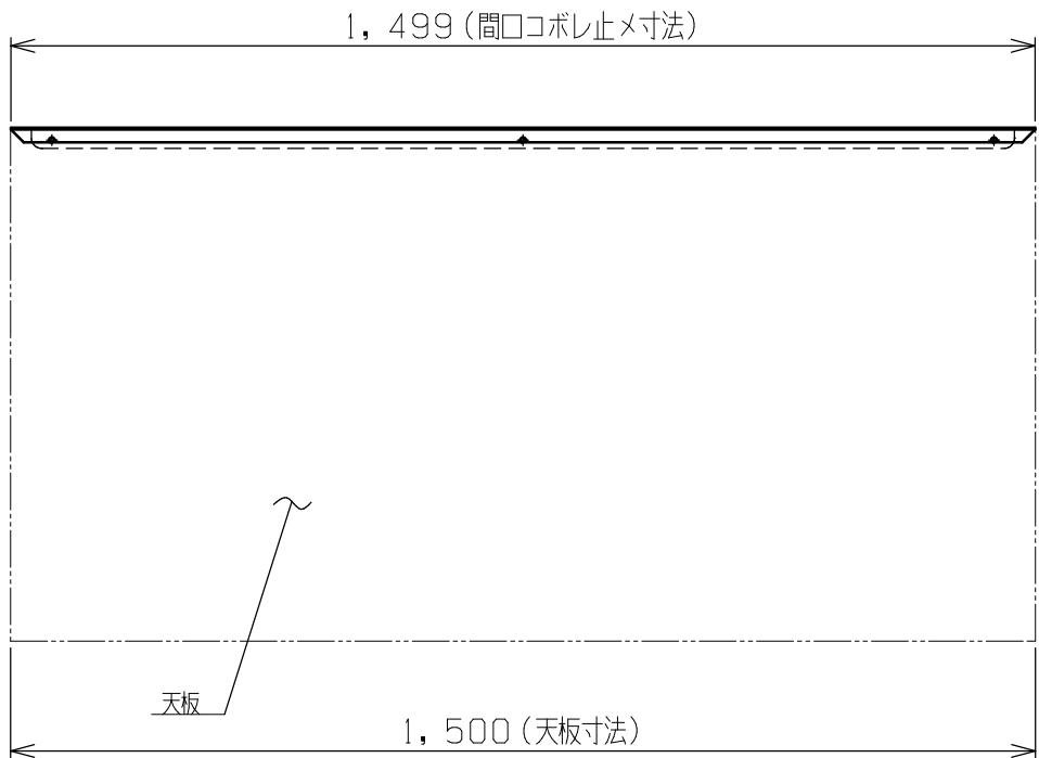
取付例 (S=1:12)
