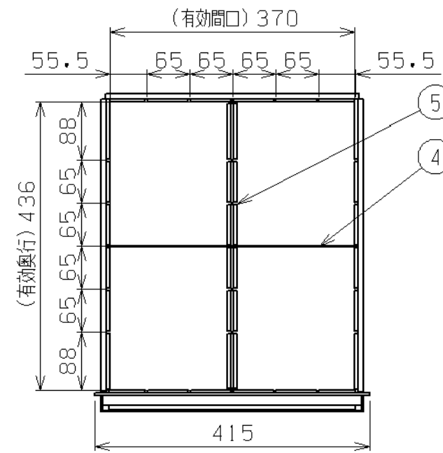
浅引出し詳細
