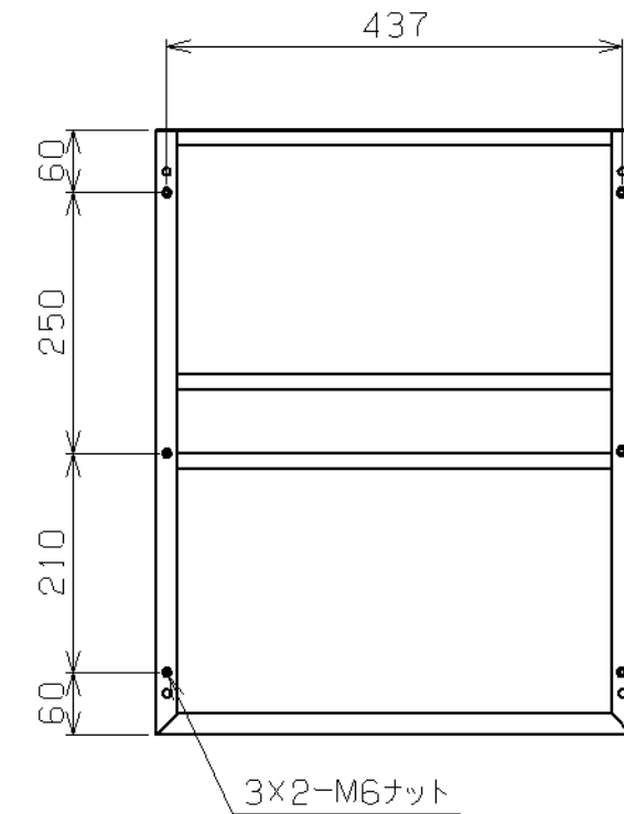
底面詳細 (矢視A)
