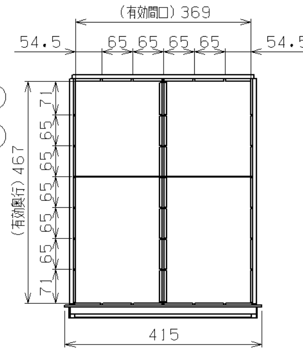
深引出し詳細
