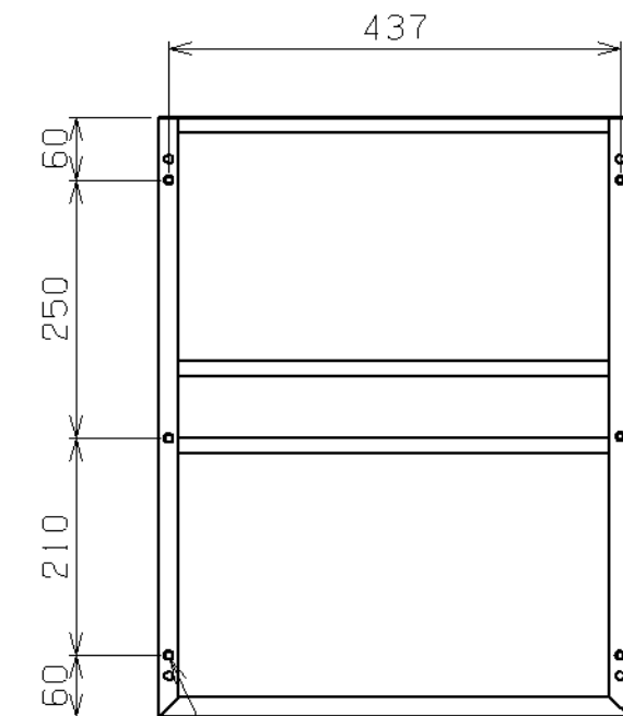
3×2-M6ナット
