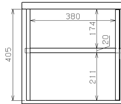
扉内詳細
