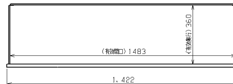
引出し詳細
