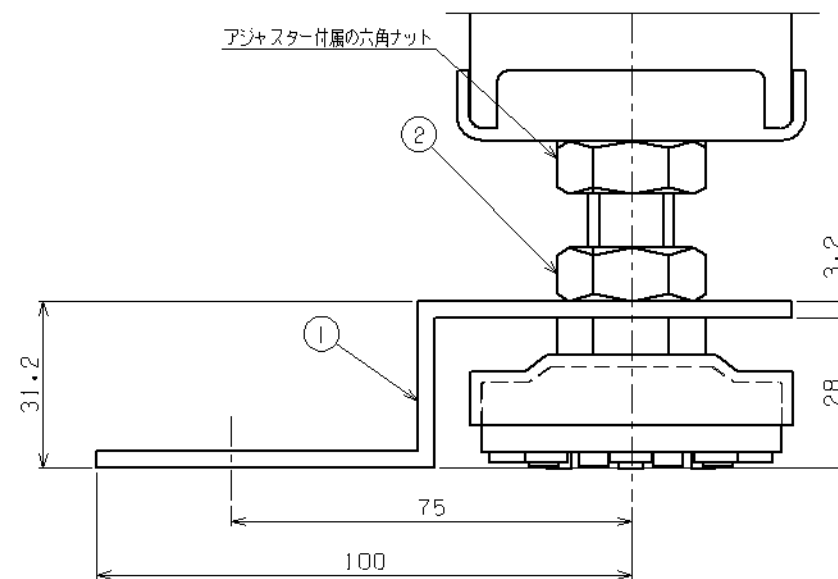
取付詳細図
