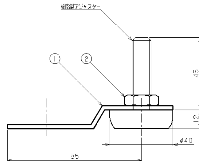
取付詳細図
