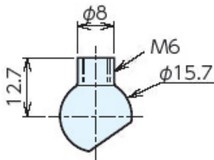
ノズル
