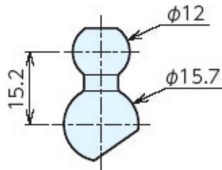
ジョイント
