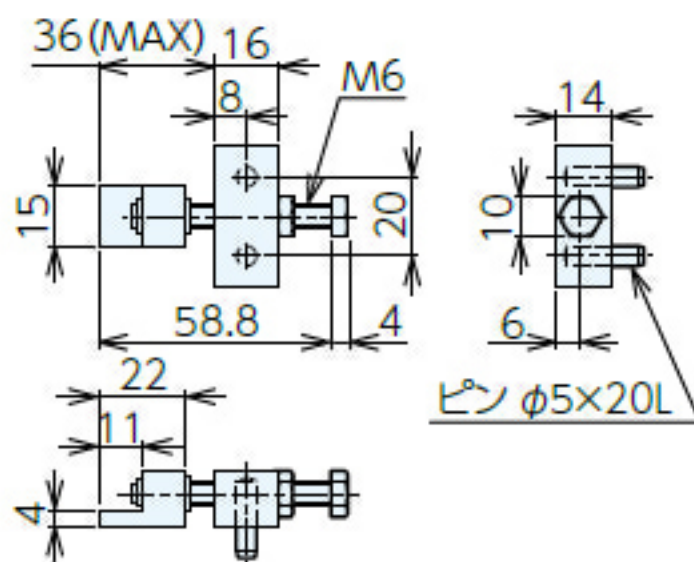
ストッパーブロックB
