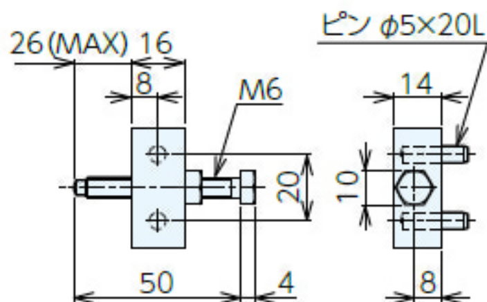
ストッパーブロックA
