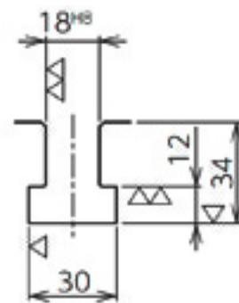
T溝詳細図
