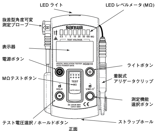
正面
