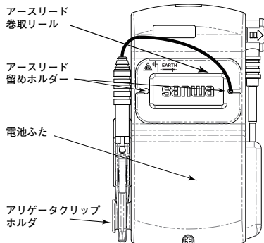
背面
