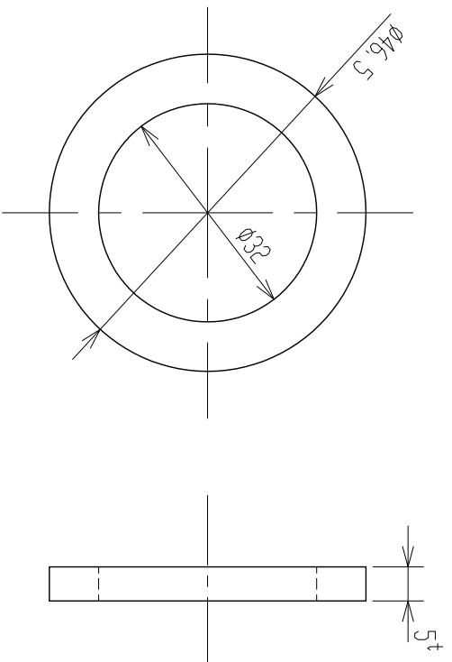
パッキン詳細 (NR)
