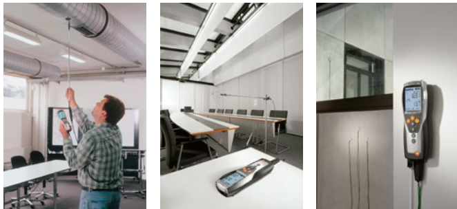
空調設備の風速・風量
