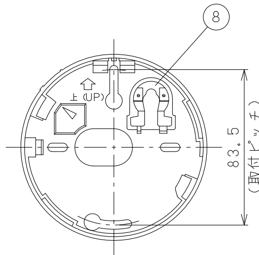
取付寸法図
