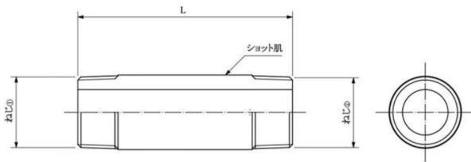
呼称30:寸法表 (mm)
