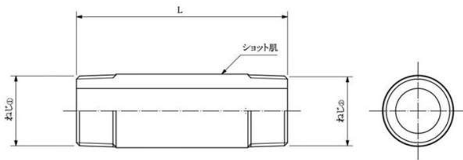
呼称25:寸法表 (mm)
