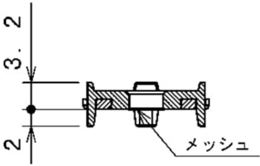
断面 A-A
