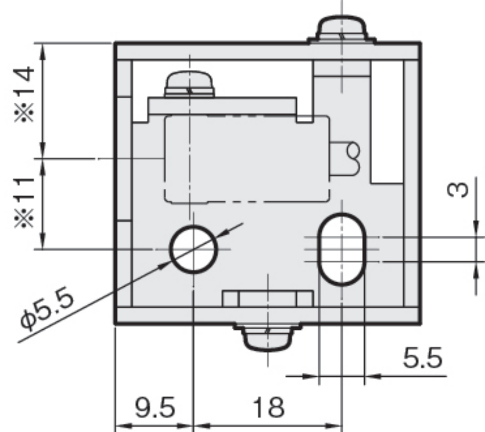
ブラケット取付穴詳細
