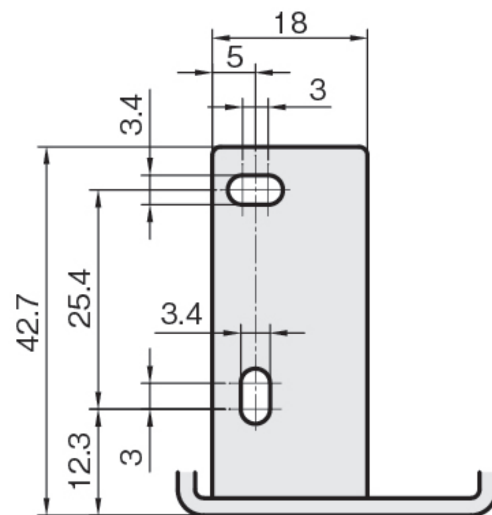
センサ取付穴詳細
