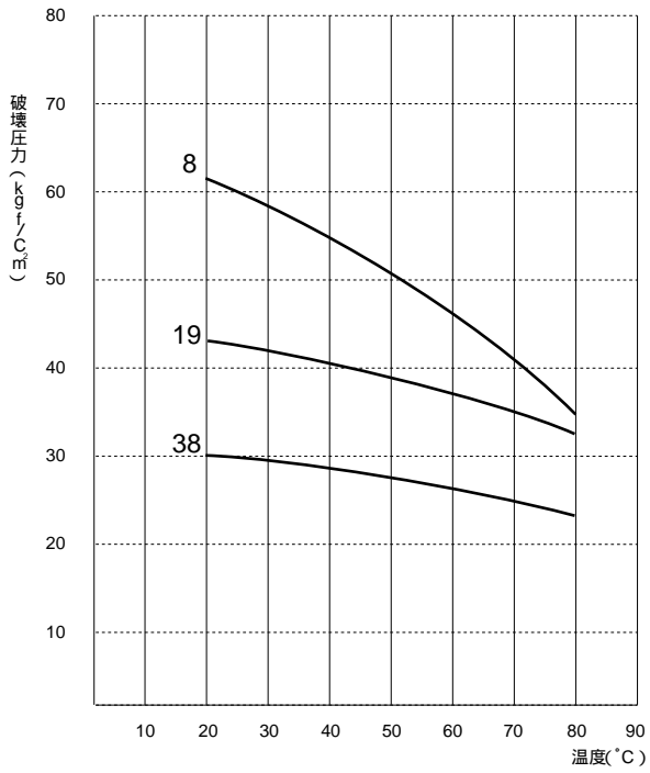
温度と破壊圧力の関係グラフ
