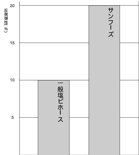
反発弾性
