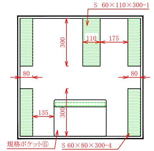
D視(後フタ)図
