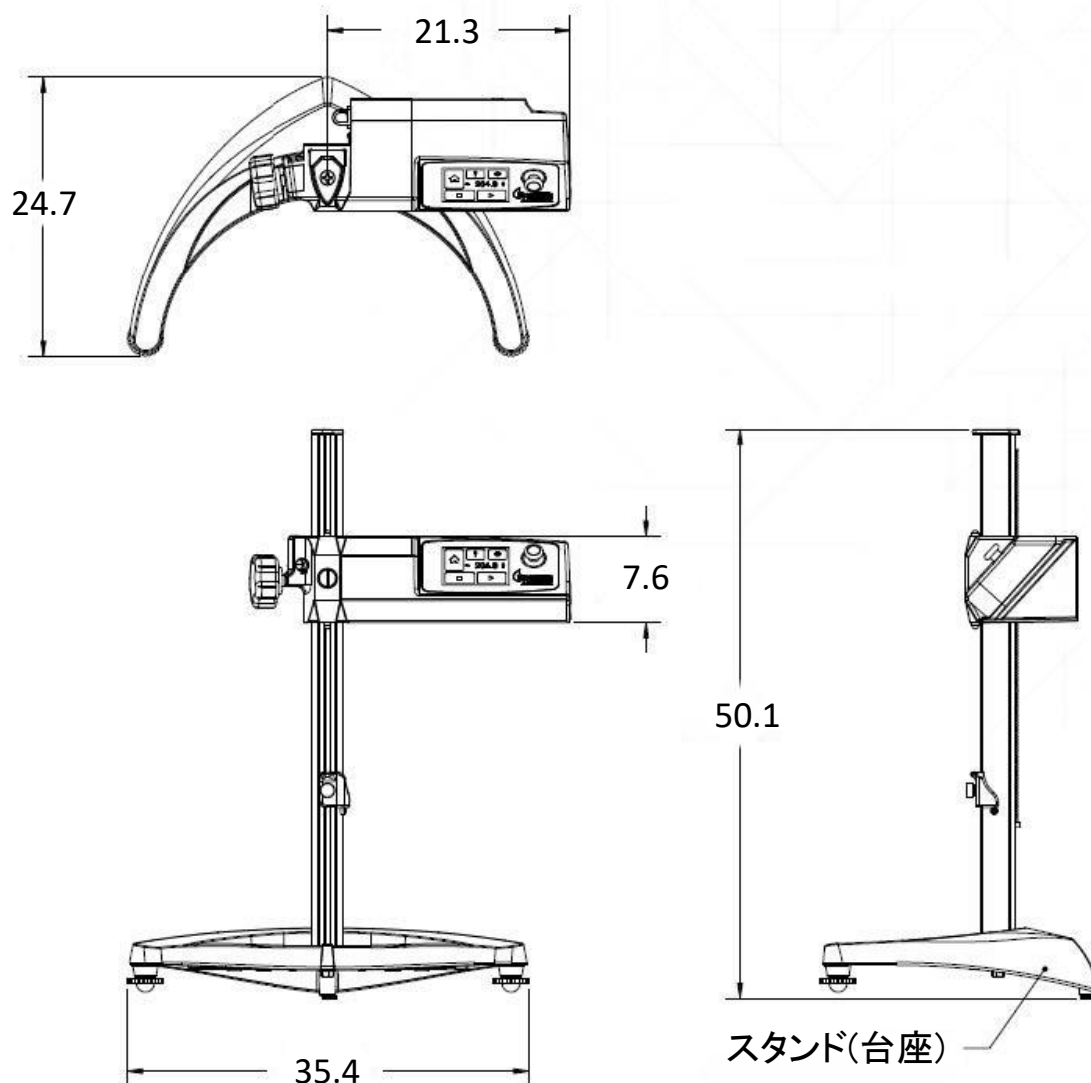
図面(外形寸法図)
