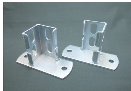
NO3 左右ストッパー金具
