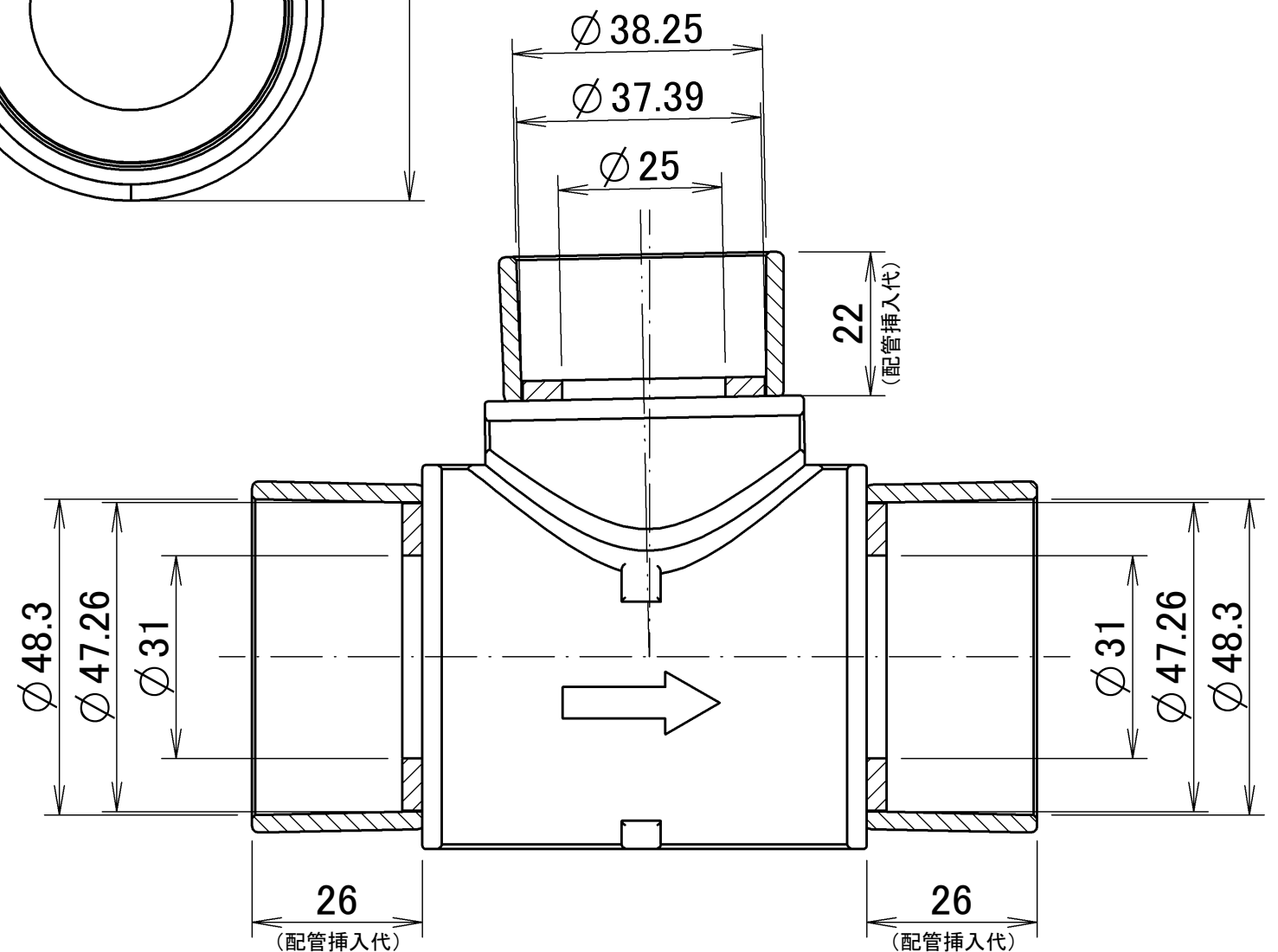
継手：受け口接合部寸法
