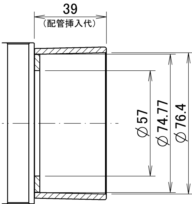
継手：受け口接合部寸法
